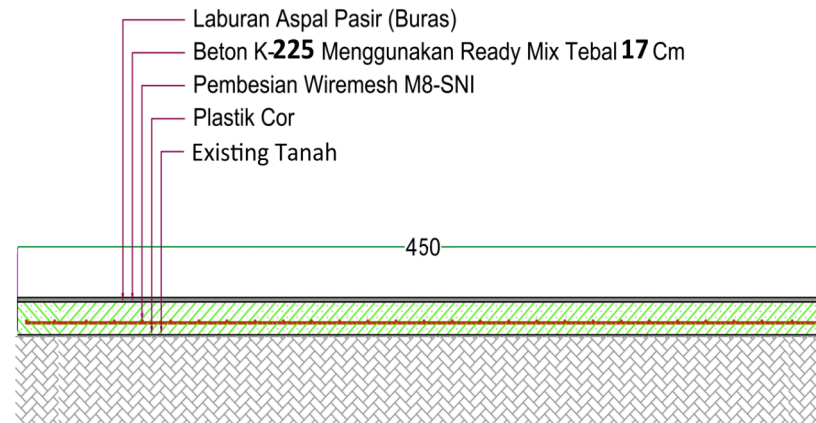
POTONGAN MELINTANG DESAIN
