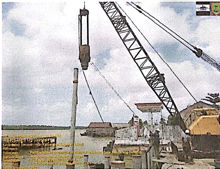
LANJUTAN PEKERJAAN PEMANCANGAN SPON PILE
