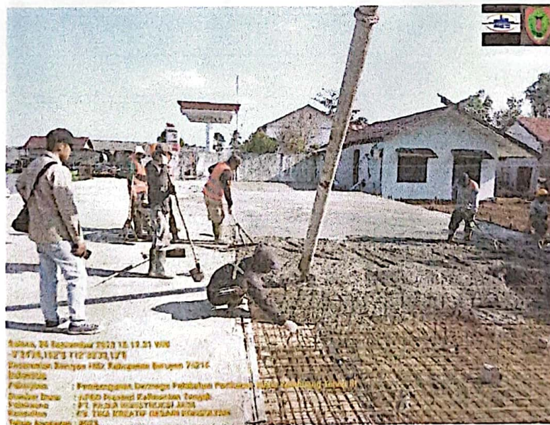
PEKERJAAN PENGECORAN SELASAR DERMAGA
