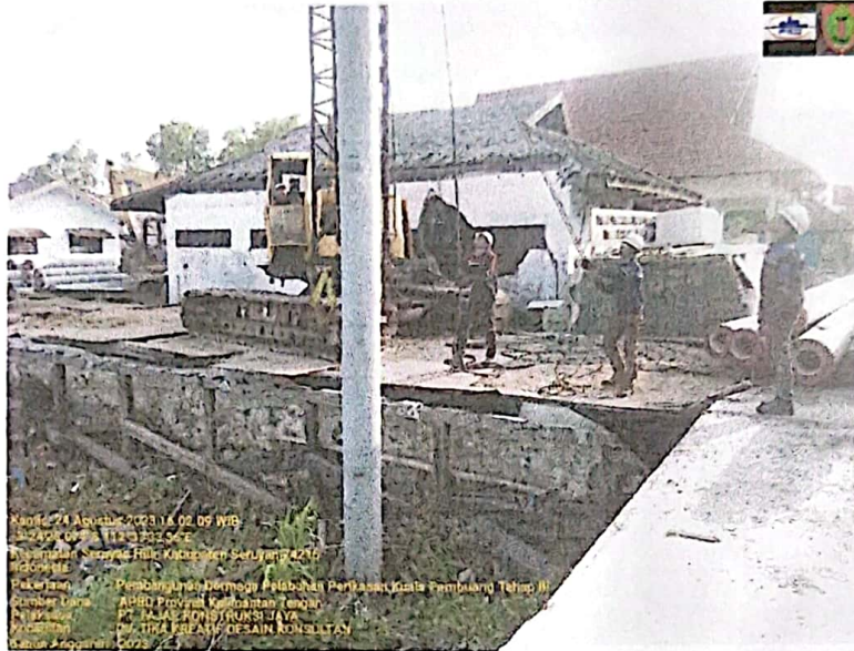
PEKERJAAN PEMANCANGAN TIANG SPON PILE TITIK PERTAMA
