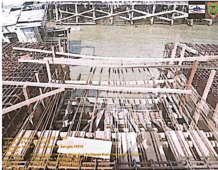
PEKERJAAN BEKISTING TANGGA
