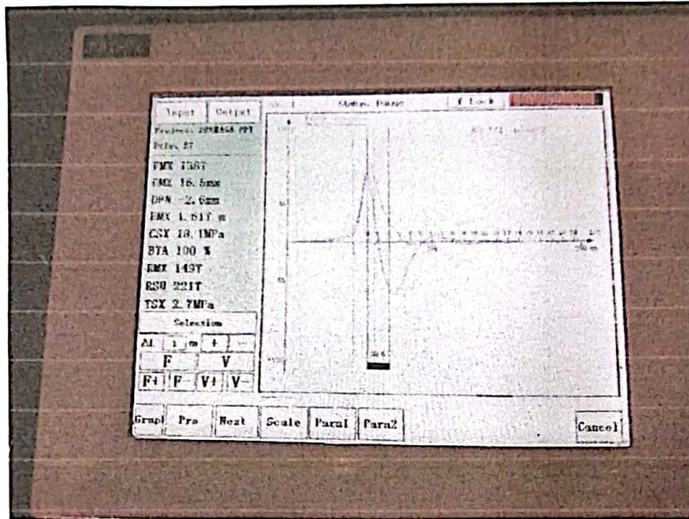
PDA TES SPON PILE 6
